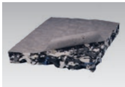
Drenážna doska pre vegetačné strechy výr. č.: 110695 Drenážna doska 25 rozmer: 1,00/2,25m
